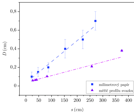
Graf 1: Závislost průměru laserového svazku D na uražené vzdálenosti s pro měření milimetrovým papírem a měřičem profilu svazku
