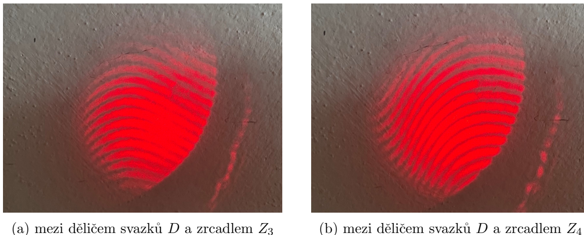
Obrázek 3: Vliv ohřátí vzduchu na interferenční obrazec
